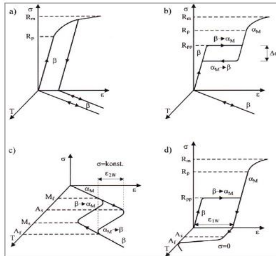
Slika 8. Ponašanje SMA materijala u uvjetima napreznja, deformacije i temperature a) ponašanje konvencionalnog materijala; b) pseudoelastičnost; c) dvosmjerni efekt; d) jednosmjerni efekt (pseudoplastičnost) 13
