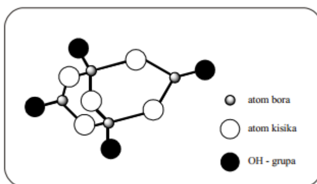
Slika 1. Struktura iona \text{B}_4\text{O}_5(\text{OH})_4^{2-}
