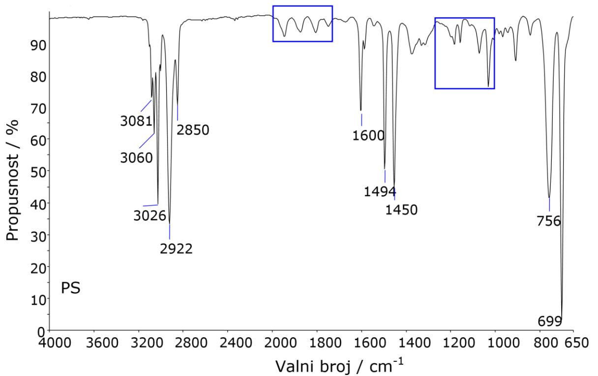
Slika 1.20. FT-IR spektar polistirena (PS). 17
