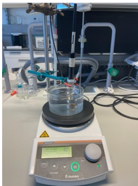
Slika 25. Aparatura za HS-SPME (Izvor: autor)
