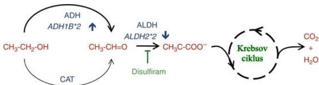
Slika 2. Metabolizam etanola. [10]
