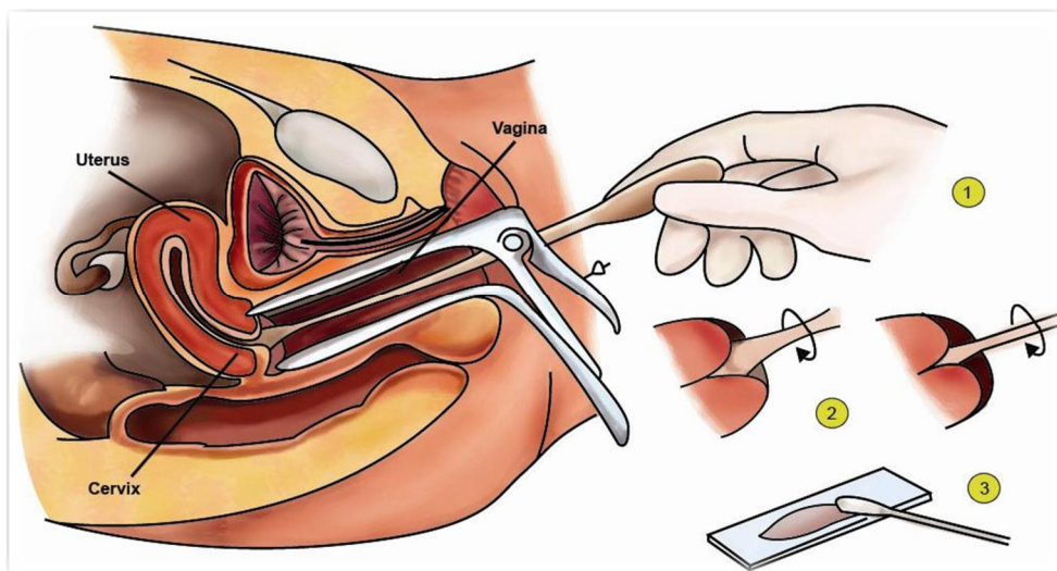
Slika 5. PAPA test
