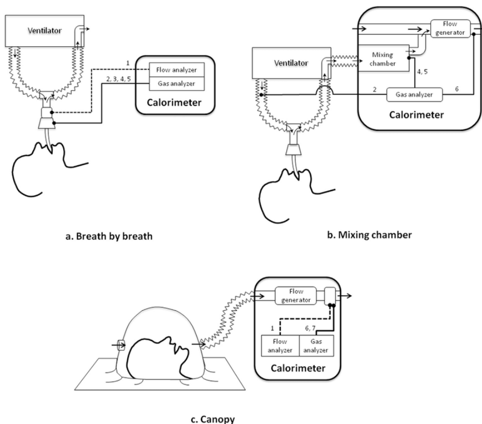
Slika 3. Prikaz izvođenja i principa indirektna kalorimetrije. Preuzeto i prilagođeno iz (11).
