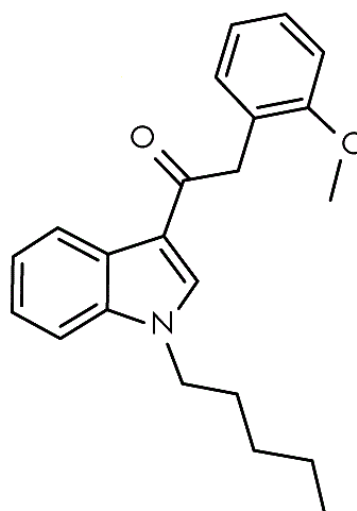
JWH-250
