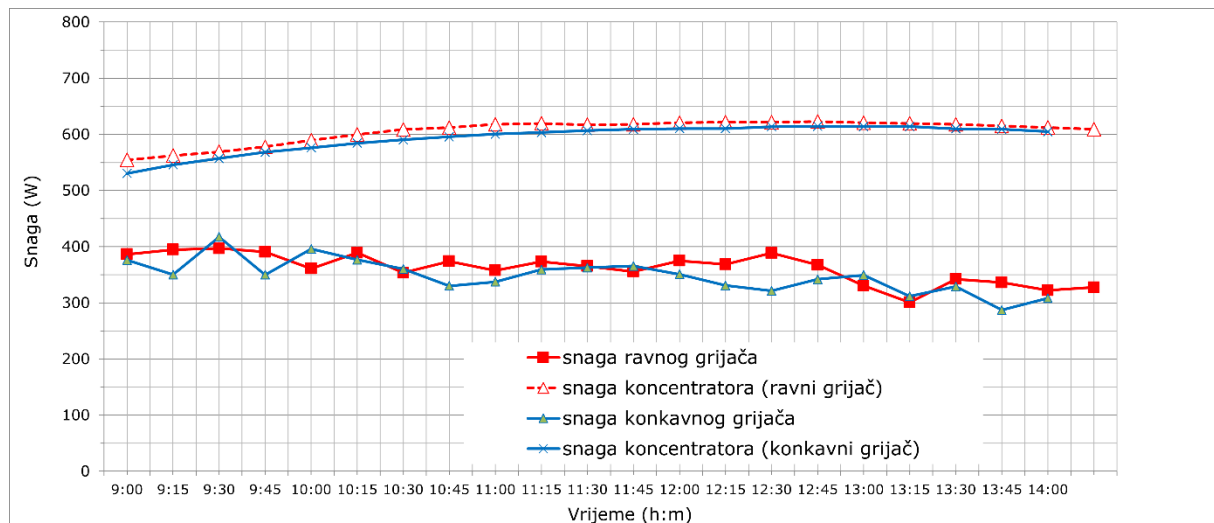
Slika 4.12. – Usporedba snage ravnog i konkavnog grijača, usporedba snage koncentrataora [3]
