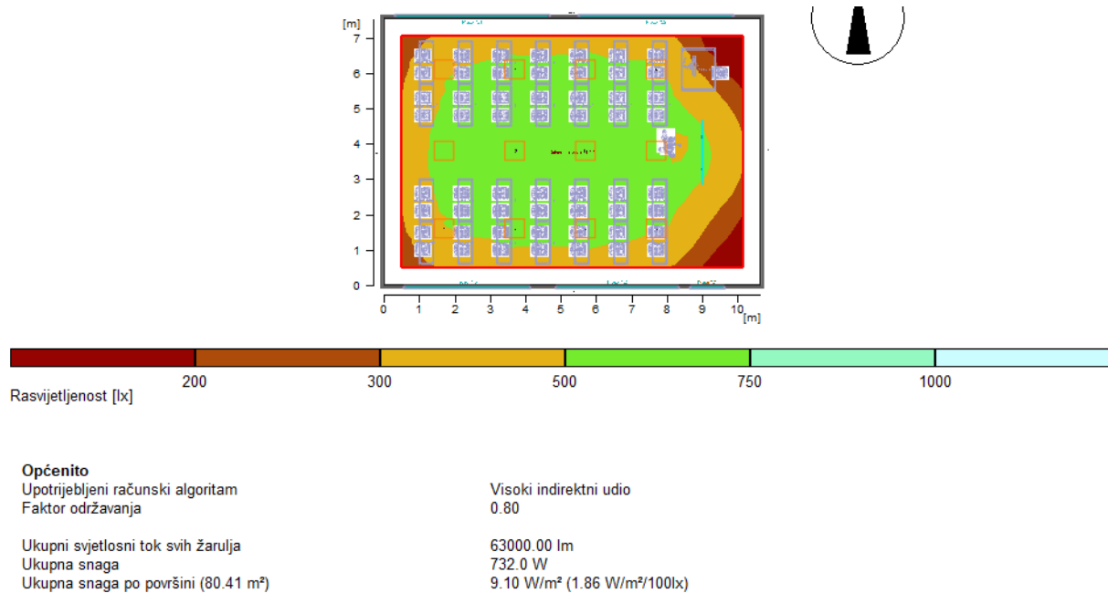
Slika 15. Rezultati proračuna postojećeg stanja predavaonice 101
