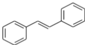
Slika 5. Osnovna kemijska struktura stilbena
