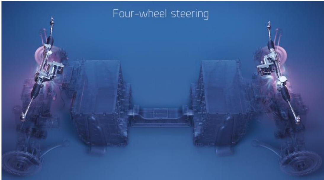
Slika 14. Izvedba kojom je omogućeno okretanje svih kotača na Zoox autonomnom vozilu
