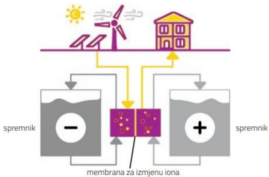
Slika 11. Prikaz djelovanja redoks protočne baterije pri pohrani električne energije iz obnovljivih izvora
