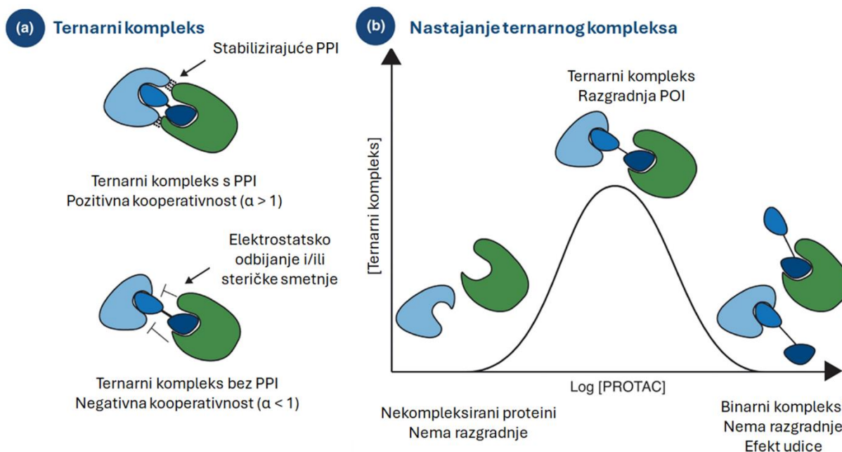
Slika 14. a) Pozitivna kooperativnost je postignuta kada su prisutne stabilizirajuće PPI između POI i E3 (gore), dok se negativna kooperativnost primjećuje kada dolazi do elektrostatskog odbijanja i/ili steričkih smetnji između POI i E3 (dolje), b) Nastajanje ternarnog kompleksa i efekt udice. POI je označen svijetloplavo, E3 ligaza zeleno, POI ligand plavo, E3 ligand tamnoplavo i poveznica crno (prilagođeno prema (62), uz licencu CC BY-NC-ND).
