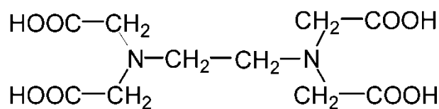
Slika 4. Struktura EDTA.
