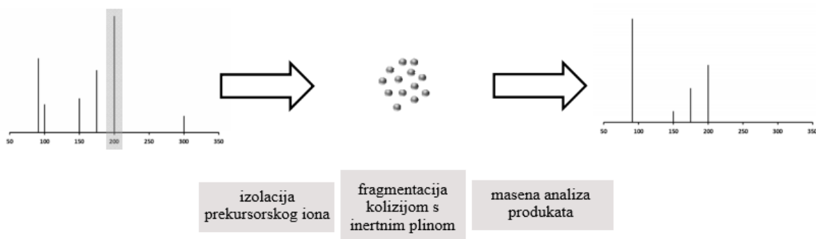
Slika 7: Princip dobivanja masenog spektra (preuzeto i prilagođeno prema Madeira i Florencio, 2012)
