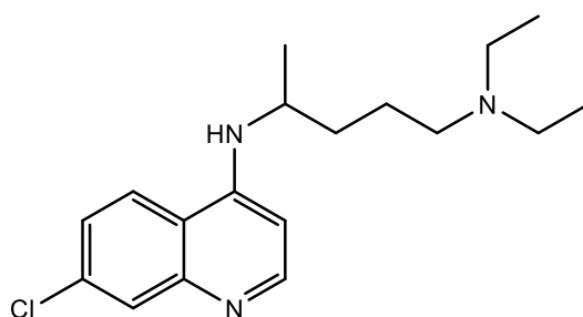
Slika 14. Struktura klorokina
