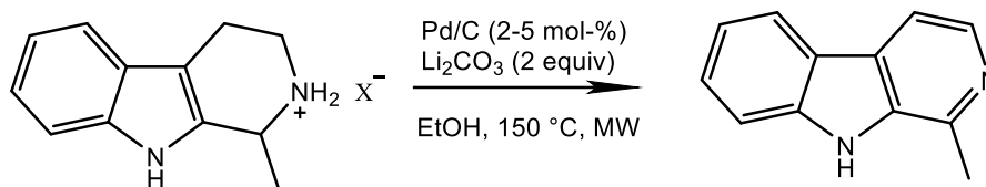
Slika 5. Aromatizacija tetrahidro- \beta -karbolina do \beta -karbolina
