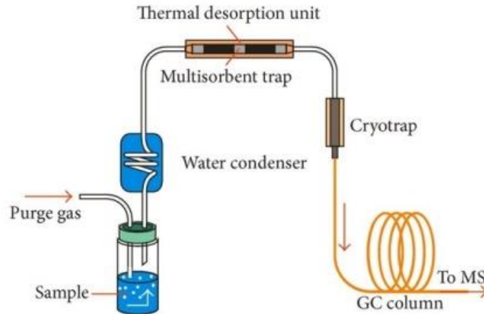
Slika 3. Shematski prikaz dinamičkog headspace uzorkovanja ( https://www.researchgate.net/ )
