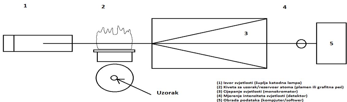
Slika 4. Shema apsorpcijskog spektrofotometra (izvor: Amidžić Klarić, 2016)
