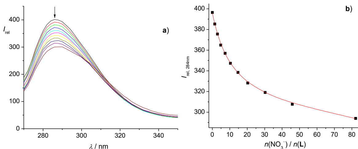
Slika 10. a) Fluorimetrijska titracija spoja L ( c = 4,57 \times 10^{-5} \text{ mol dm}^{-3} ) s \text{TBANO}_3 ( c = 9,09 \times 10^{-3} \text{ mol dm}^{-3} ) u acetonitrilu pri 25 °C. \lambda_{\text{ex}} = 260 \text{ nm} , eksitacijski prorez = 10 nm, emisijski prorez = 10 nm. b) Ovisnost relativnog intenziteta fluorescencije o množinskom omjeru n(\text{NO}_3^-) / n(\text{L}) . ■ izmjerene vrijednosti; — izračunate vrijednosti.
