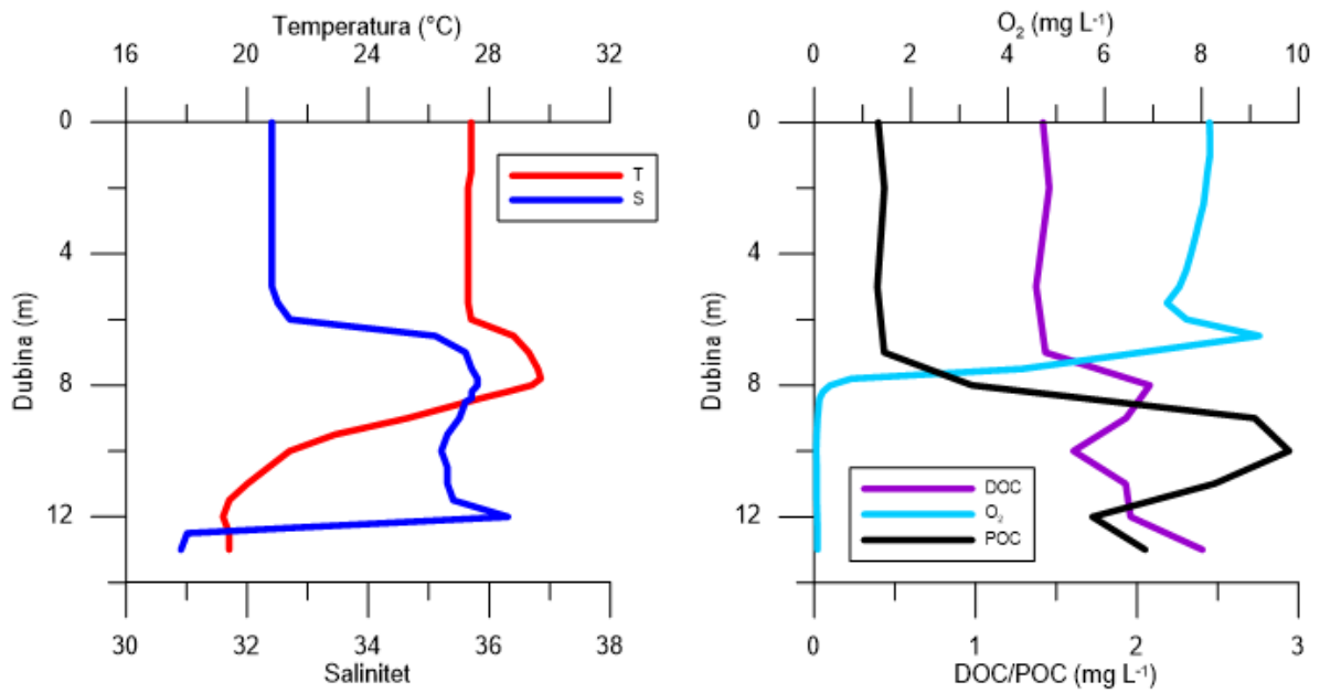
Slika 26. Vertikalni profili vodenog stupca jezera Zmajevo oko na dan 26. kolovoza 2013. Koncentracija otopljenog kisika (O 2 ), koncentracija otopljenje organske tvari (DOC), koncentracija čestične organske tvari (POC).
