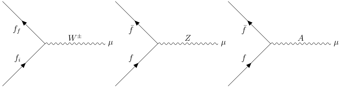
Slika A.2: Fermion-bozon-fermion međudjelovanja u elektroslaboј teoriji prema izrazima (A.13), (A.18) i (A.19).
