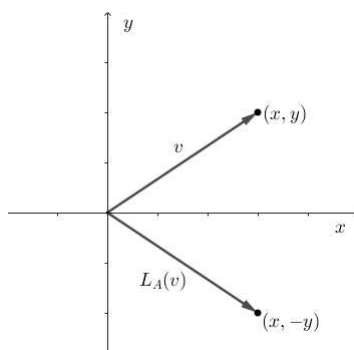
Slika 1.6: Očna simetrija s obzirom na x -os
