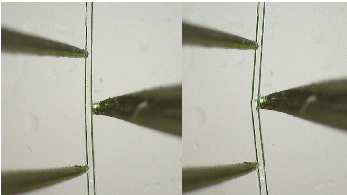
Slika 37. Postupak savijanja kristala spoja [\text{Zn}(\text{SCN})_2(\text{nia})_2] (3) i njegovo pucanje, pod mikroskopskim povećanjem od 50 puta.
