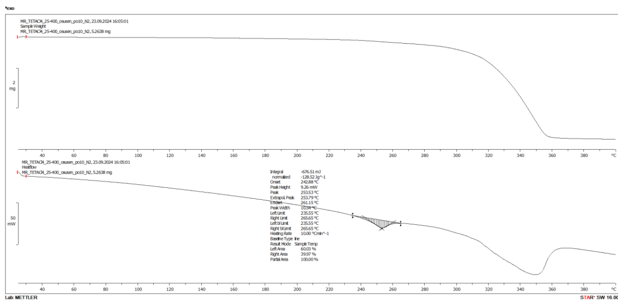
Slika D13. TG/DSC krivulja pripravljene kloridne soli trietilentetraamina: (H 4 TETA)Cl 4 .
