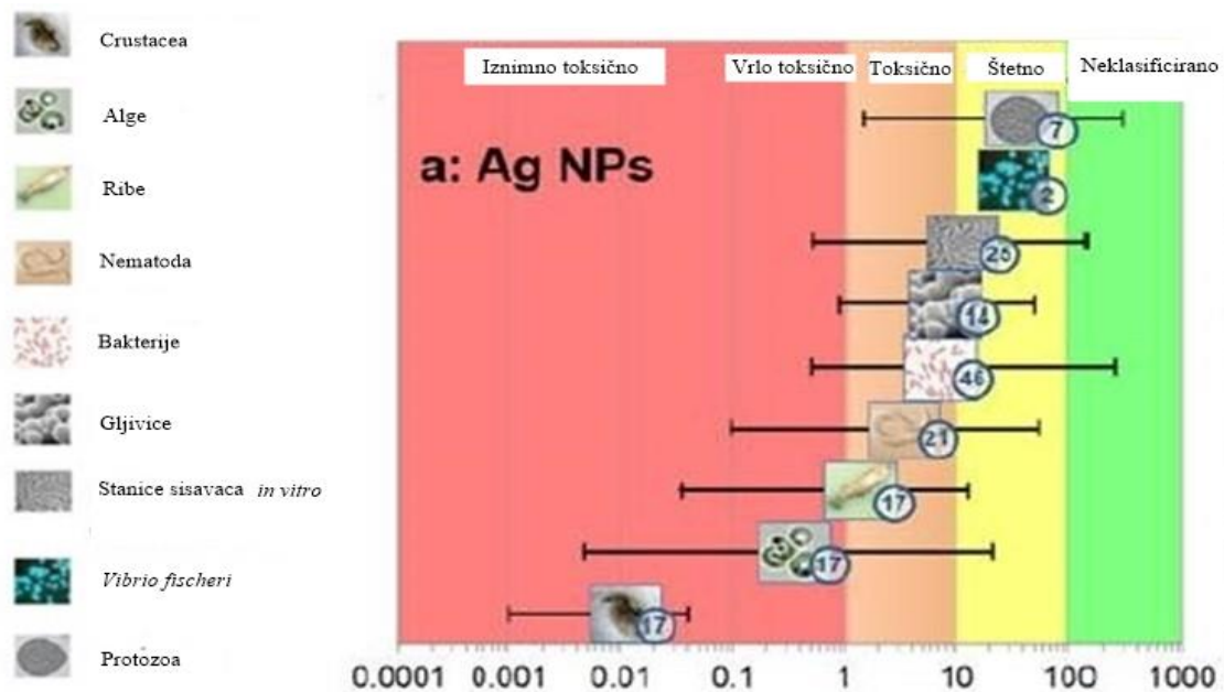
Slika 24. Piktogram medijana EC_{50} vrijednosti \pm minimalne i maksimalne vrijednosti (iz većeg broja istraživanja) za testne vrste s pripadajućom legendom. Na x-osi su koncentracije nanosrebra u mg Ag/L. Različite boje unutar piktograma predstavljaju kategorizaciju toksičnosti prema EU-Direktivi 93/67/EEC (preuzeto i prilagođeno iz Bondarenko i sur., 2013.).
