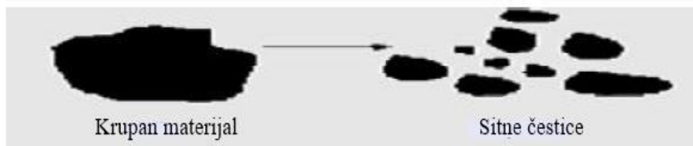
Slika 9. Shematski prikaz „ top-down “ metode (preuzeto i prilagođeno iz Singh i sur., 2010).
