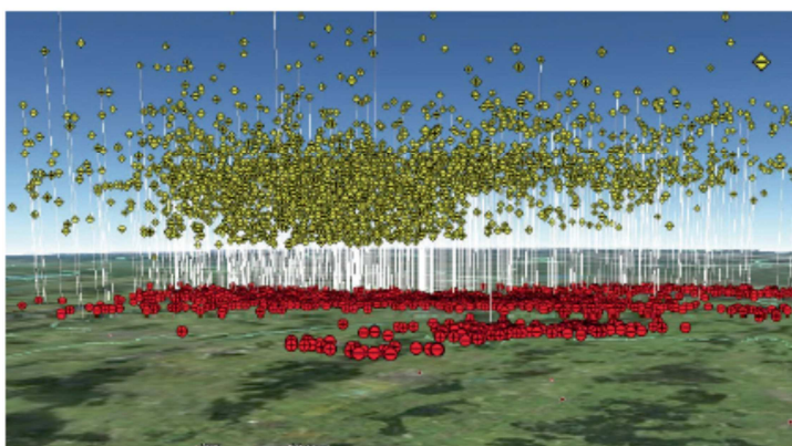
Slika 48: 3D prikaz oluje koja se približavala Münchenu 7. 7. 2007. U vremenu od 17 do 18 UTC. Prikaz je dobiven LINET sustavom. Žuto su prikazane munje u oblaku, a crveno munje oblak – zemlja. Broj munja u oblaku bio je 4 puta veći nego broj munja oblak – zemlja što pokazuje veliku elektriziranost oblaka tj. veliki grmljavinski sustav. [8.]
