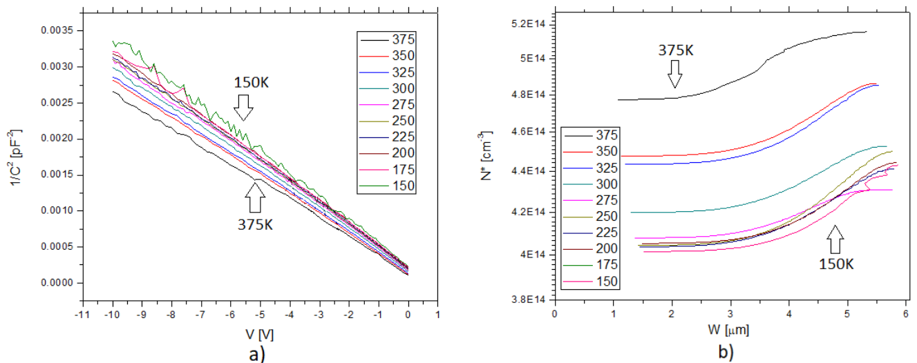
Slika 17: a) Graf 1/C^2 vs. V za različite temperature, b) Dubinsko profiliranje koncentracije slobodnih nosilaca na različitim temperaturama, Si dioda
