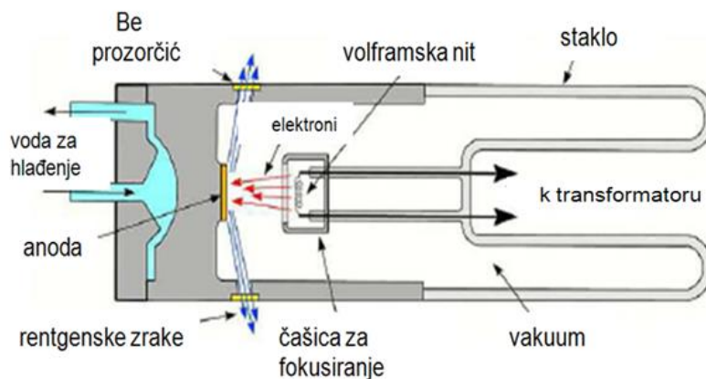
Slika 34. Shematski prikaz rendgenske cijevi 19
