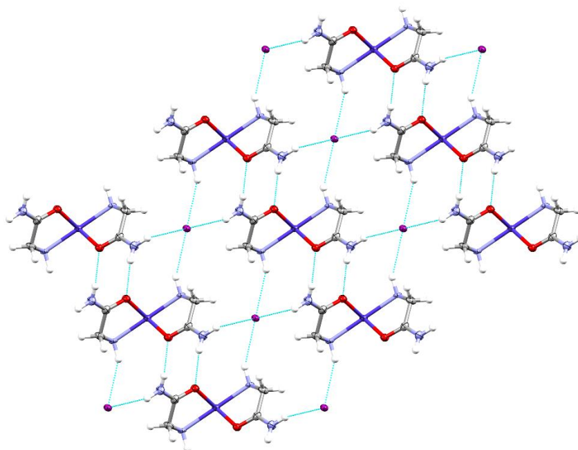
Slika 51. Vodikove veze spoja [\text{Co}(\text{idaa})_2]\text{I}_3\text{I} u ravni (010) (za izradu crteža upotrebljen je program Mercury 3.8. ) 16
