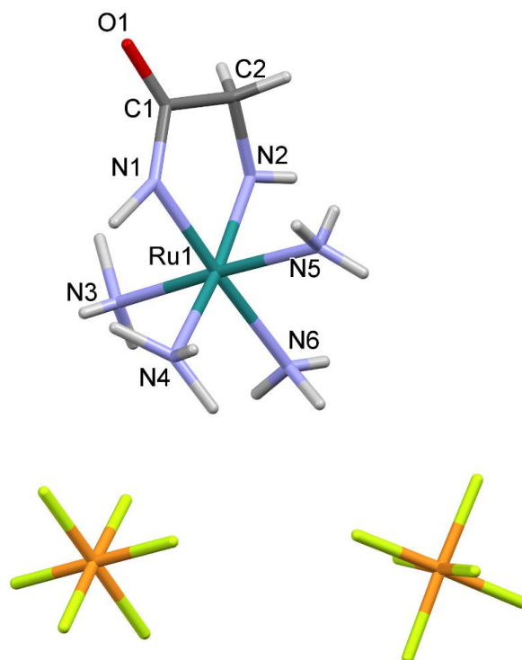
Slika 16. Kristalna struktura [\text{Ru}(\text{Glyam})(\text{NH}_3)_4](\text{PF}_6)_2 ( refcode : DOXDID) (za izradu crteža upotrebljen je program Mercury 3.8. ) 16
