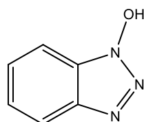
hidroksibenzotriazol HOBt
