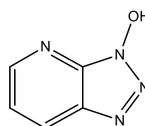
1-hidroksi-7-azabenzotriazol HOAt
