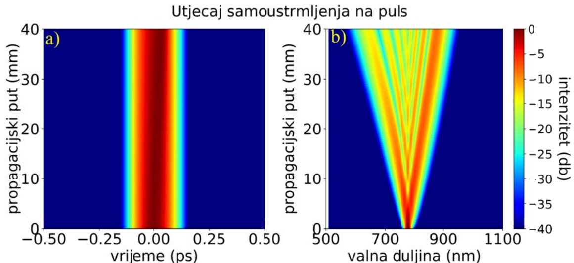
Slika 3.18: Utjecaj samoustrmljenja na puls. Slika a) Vremensku evolucija pulsa. Vrh pulsa se zbog različitih grupnih brzina vrha i rubova pulsa počinje naginjati prema pratećem krilu pulsa te puls prestaje biti simetričan. Slika b) Utjecaj samoustrmljenja na spektar pulsa. Parametri optičkog vlakna: \beta_2 = 0 \frac{ps^2}{km} , \beta_3 = 0.0 \frac{ps^3}{km} , \gamma = 70 \frac{1}{Wkm} za vlakno duljine L=4 cm.
