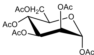
Slika 9. Strukturna formula spoja 5
