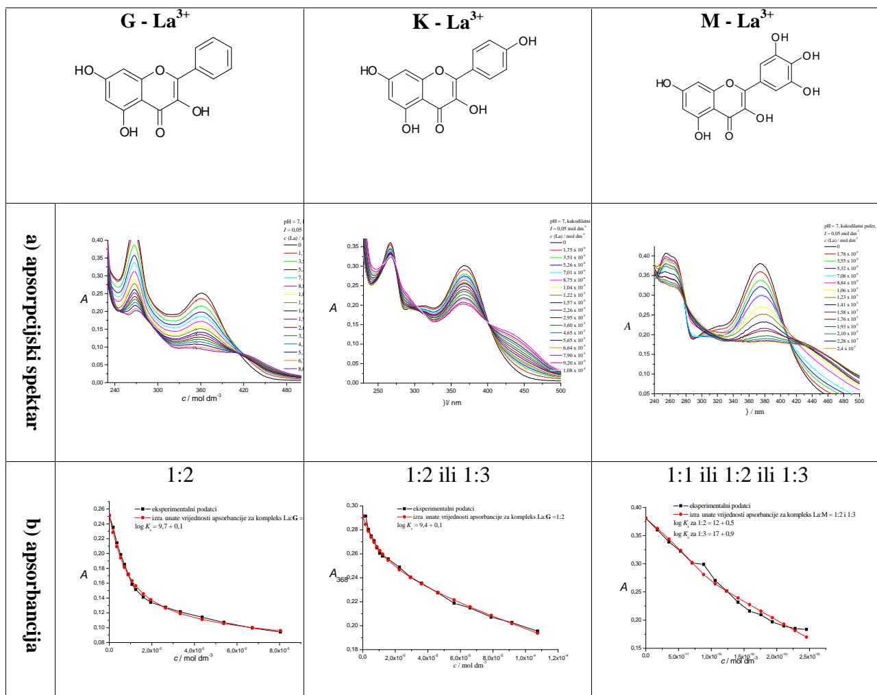
Tablica 7. a) Promjene UV/Vis spektara G , K i M nakon dodatka vodene otopine lantana(III) ( c = 1,8 \times 10^{-3} \text{ mol dm}^{-3} ), u kakovodilatom puferu ( \text{pH} = 7 , I = 0,05 \text{ mol dm}^{-3} ), c(\text{G, K ili M}) = 2,0 \times 10^{-5} \text{ mol dm}^{-3} ; b) utjecaj promjene koncentracije lantana(III) na eksperimentalne i izračunate vrijednosti apsorpcije G , K i M za model stehiometrije \text{La(III)-flavonoid}=1:2 .
