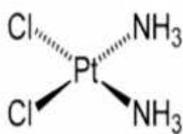
Slika 6. Molekula cisplatine
