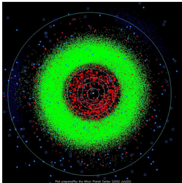
Slika 1. Prikaz raspodjele asteroida u Sunčevu sustavu – elipse predstavljaju orbite planeta; zeleno su prikazani asteroidi Glavnog asteroidnog pojasa; crveno su prikazani asteroidi koji izlaze iz Glavnog asteroidnog pojasa te se zbog gravitacijskih sila mogu sudariti sa Zemljom
