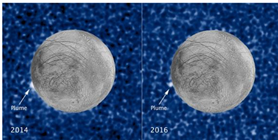
Slika 17. Prikaz izbacivanja oblaka vodene pare s istog mjesta na površini mjeseца Europe u razmaku od dvije godine snimljen teleskopom Hubble pod UV svjetlom (17. ožujka 2014. – lijevo, 14. veljače 2016. – desno)
