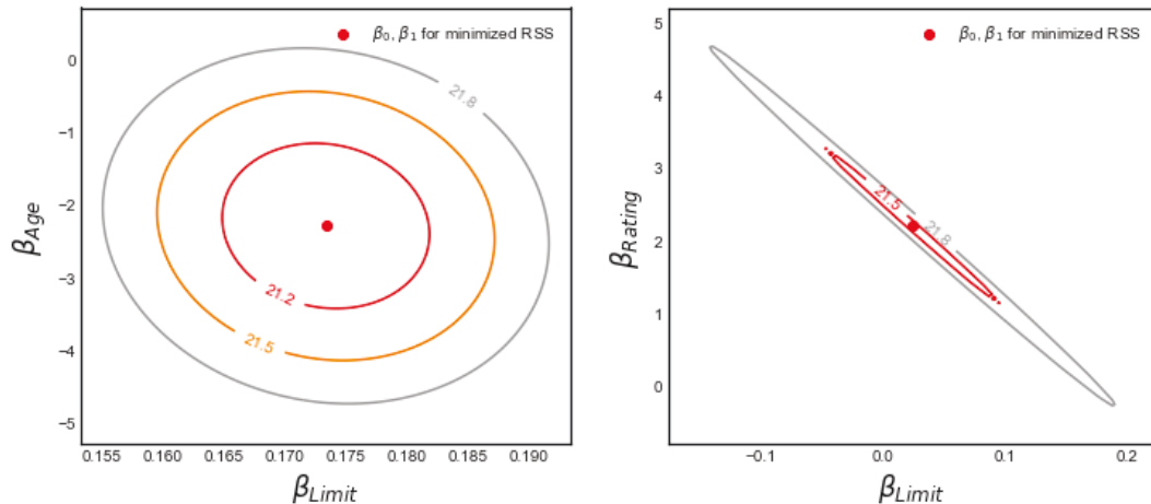
Slika 3.2: "Contour plot" za različite vrijednosti RSS prikazanih preko funkcijske ovisnosti o koeficijentima predikcije \beta . Crvenom točkom prikazana je najmanja vrijednost za RSS [10].
