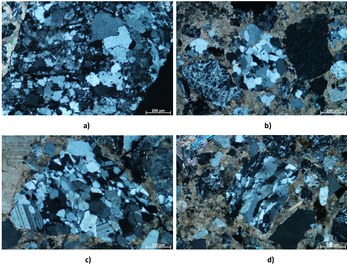
Slika 5.7: Litoklasti granitoida i nekih metamornih stijena (kvarcni i kvarcno-feldspatski protoliti) u konglomeratima; a) mikrogranit (N+); b) kvarcit (N+); c) granofels (Ab + Qtz). U gornjem dijelu zrna zapaža se pojava lećastog "uslojavanja" kvarca ( lenticular compositional layering ) (N+); d) deformirani agregat kvarca s vidljivim "podzrnima" ( subgrains ) unutar pojedinih kvarcnih zrna u agregatu (N+).
