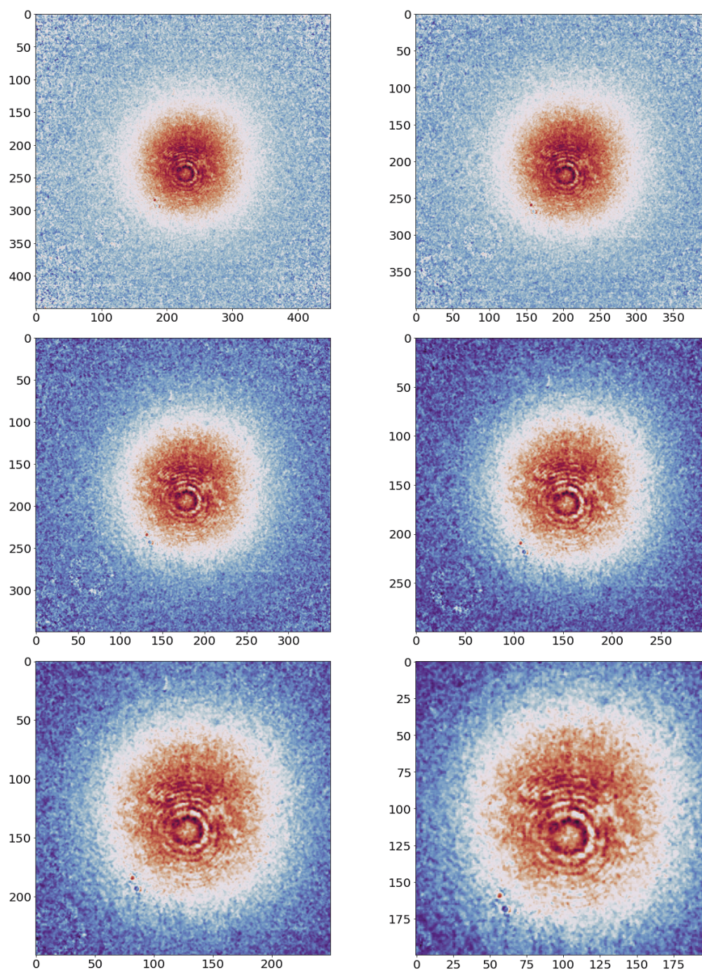
Slika B.1: Oblak atoma za različite rezolucije slike. TOF= 10ms, t_{load} = 4.25s .
