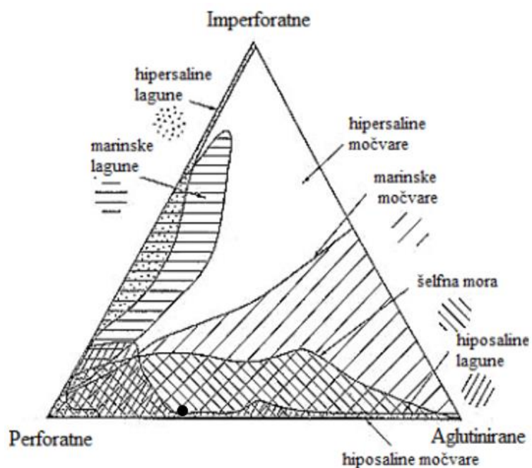
Slika 15 Prikaz trokomponentnog dijagrama za određivanje okoliša s obzirom na tip stijenki za uzorak K4 (modificirano prema Murray, 1974)
