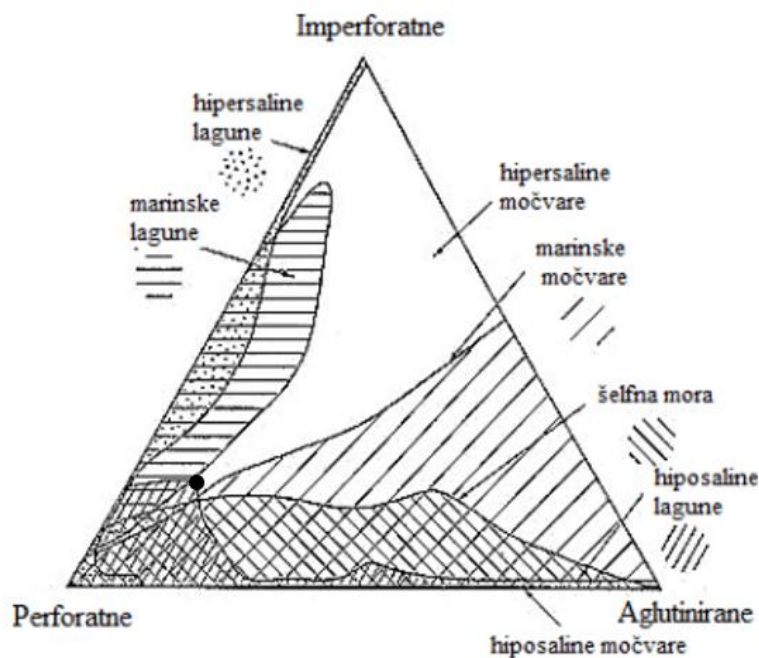
Slika 16 Prikaz trokomponentnog dijagrama za određivanje okoliša s obzirom na tip stijenke za uzorak K6 (modificirano prema Murray, 1974)
