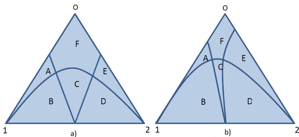
Slika 3. Primjeri izoternnih ternarnih dijagrama pod a) sličnih topljivosti koformera 1 i 2 u otapalu O i pod b) različiti topljivosti koformera 1 i 2 u otapalu O. Regije u dijagramu: A, koformer 1 i otopina; B, koformer 1 i kokristal; C, kokristal; D, koformer 2 i kokristal; E, koformer 2 i otopina; F, otapalo. 7
