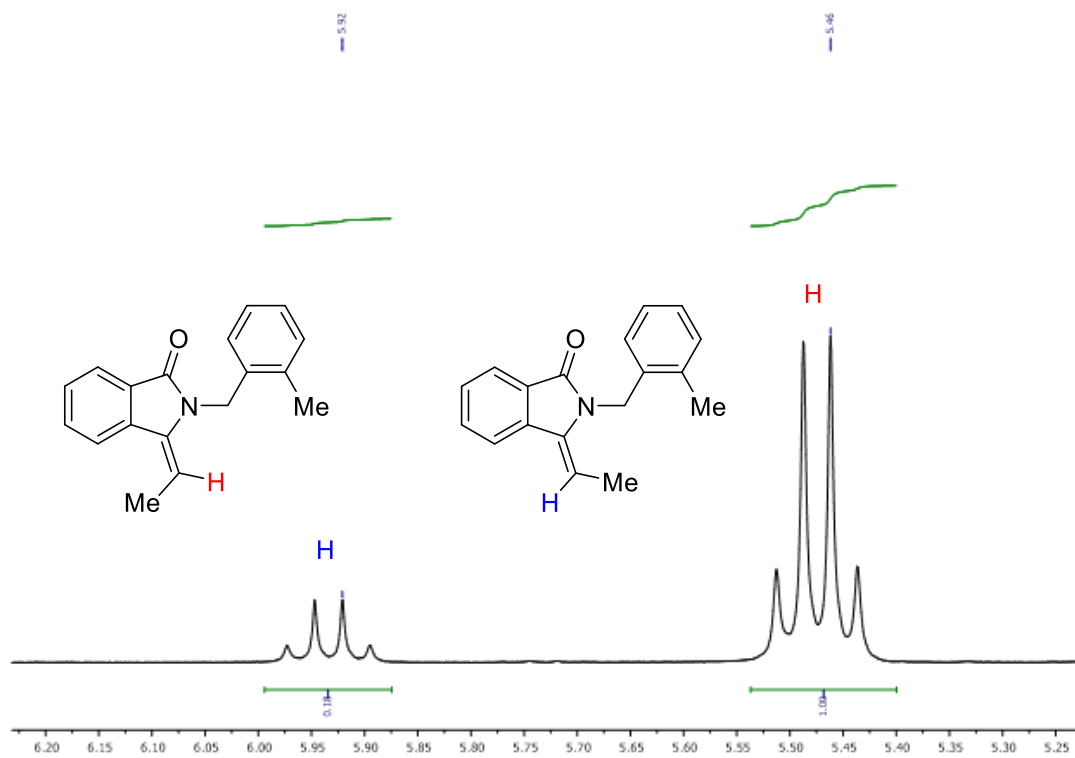
Slika D58. Segment 1 H NMR spektra spoja 2i
