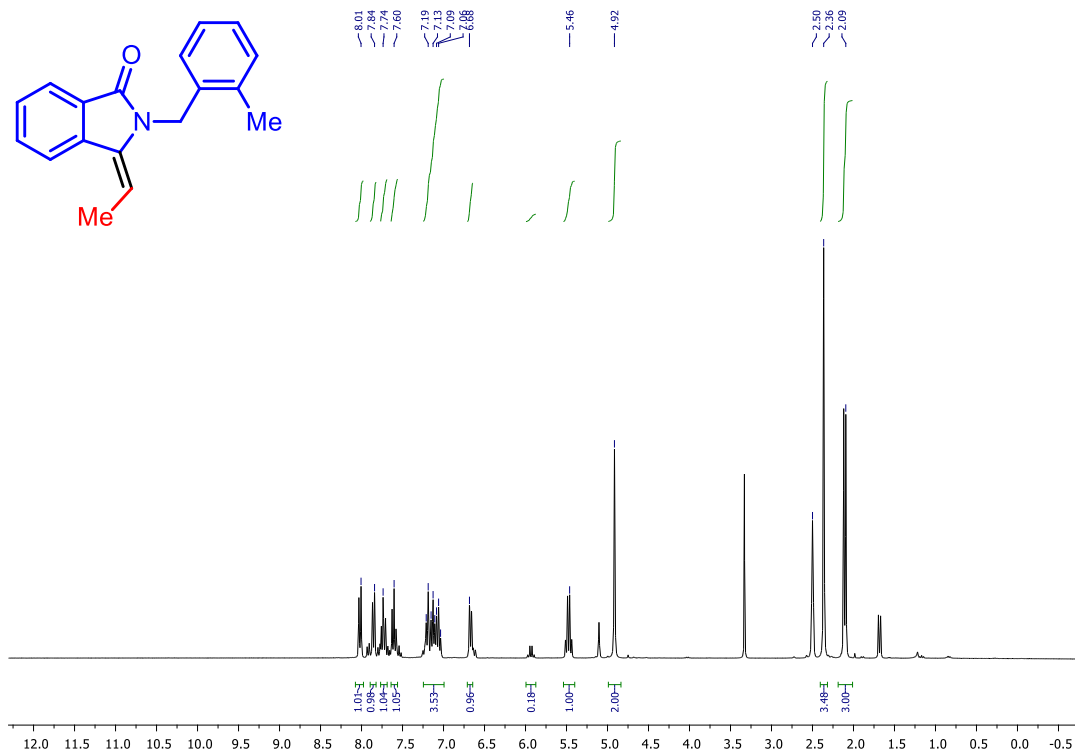
Slika D57. 1 H NMR spektr ( E )-3-etiliden-2-(2-metilbenzil)izoindolinona ( E -2i)
