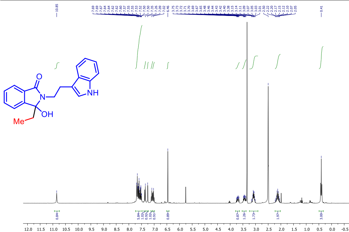
Slika D32. ^1\text{H} NMR spektar 2-(2-(1H-Indol-3-il)etil)-3-etil-3-hidroksiizindolinona ( 1z )
