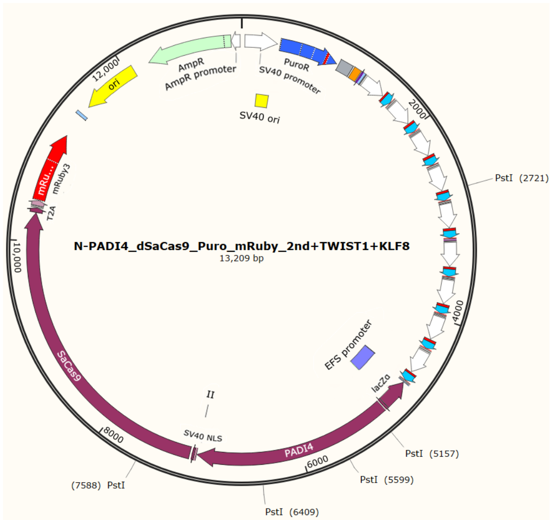
Slika 26. Završni PAD4-dCas9 fuzijski konstrukt s devet različitim molekulama sgrRNA za istovremeno ciljanje genskih lokusa TWIST1 i KLF8 . Naznačena su restrikcijska mjesta PstI korištena za provjeru konstrukta restrikcijskom analizom.
