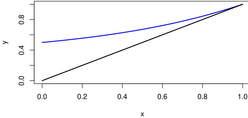
Slika 2.4: Prikaz funkcije izvodnice sub-kritične distribucije potomaka
