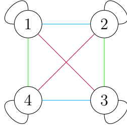
Slika 7: asocijacijska shema dobivena od klasa konjugacije grupe (\mathbb{Z}_2 \times \mathbb{Z}_2, +) reprezentirana pomoću obojanog grafa i pripadne matrice
