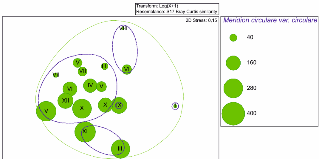
Slika 20. Sezonska zastupljenost vrste Meridion circolare var. circularis .
