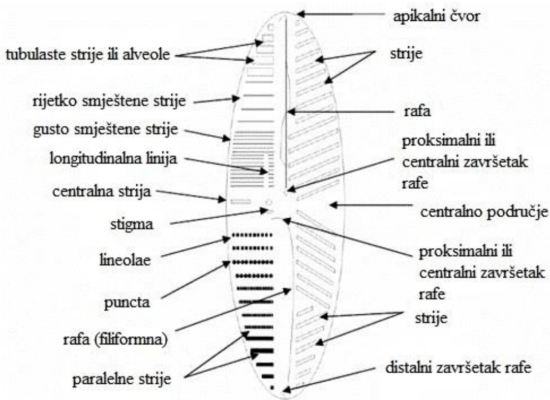
Slika 4. Glavne morfološke karakteristike ljuštare alge kremenjašice s bilateralnom simetrijom.
