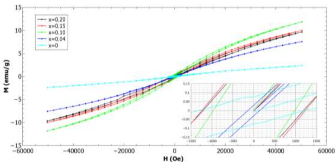
Slika 5.1: Krivulja magnetske histereze za YMn_{1-x}Ti_xO_3 pri T = 3 K. Na umetku je uvećano prikazan dio oko malih polja.
