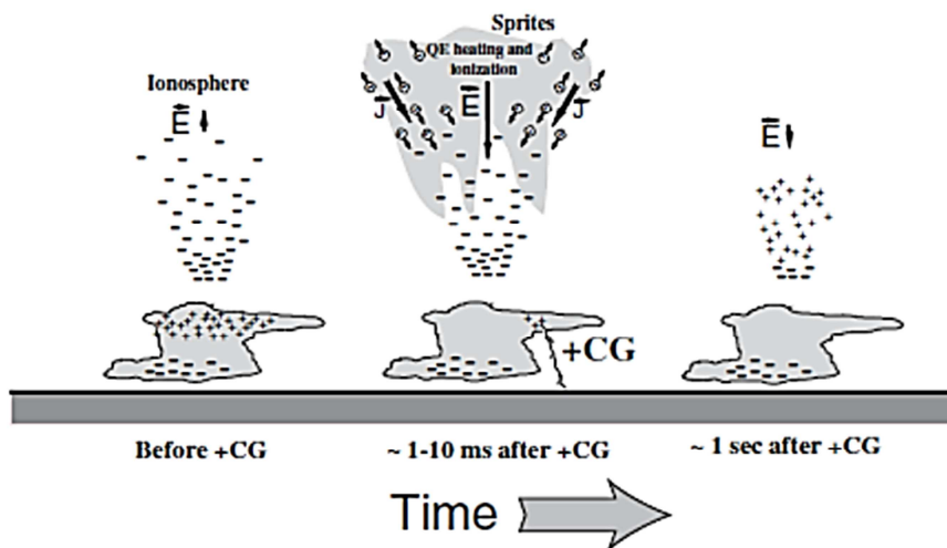
Slika 33: Prikaz mehanizma prodiranja velikog električnog polja do mezosfere i formiranja vilenjaka [9.]
