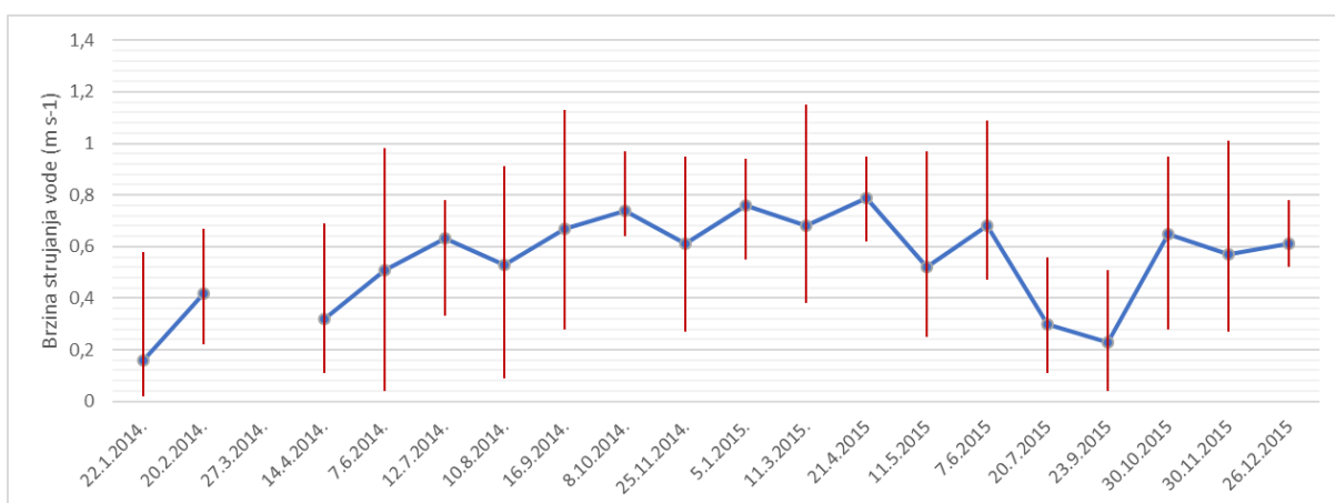
Slika 16. Prosječna brzina strujanja vode ( \text{m s}^{-1} ) (plava linija) s rasponom (min-maks) izmjerena u Tonkovića vrilu u razdoblju od siječnja 2014. godine do prosinca 2015. godine.
