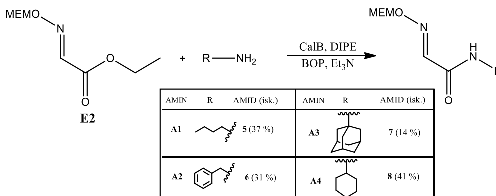
Slika 50. Reakcije estera etil-MEM-gliksilat oksima E2 provedene CalB-BOP metodom s aminima: n -butilaminom A1 , benzilaminom A2 , 1-adamantilaminom A3 i cikloheksilaminom A4
