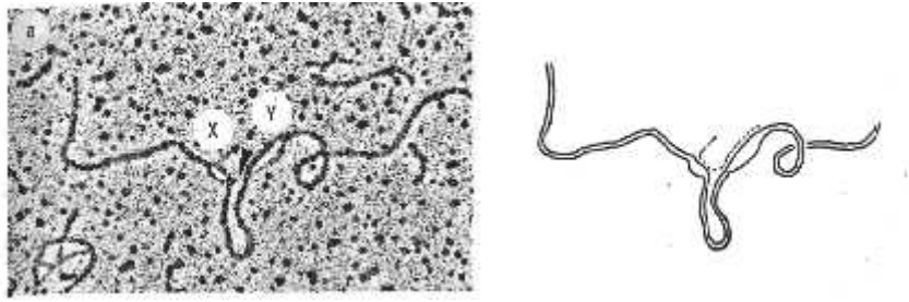
Slika 6. Slika snimljena elektronskim mikroskopom na kojoj je vidljivo stvaranje omotača na dijelu DNA koji se nije sparilo s komplementarnom mRNA (Chow i suradnici, 1977).
